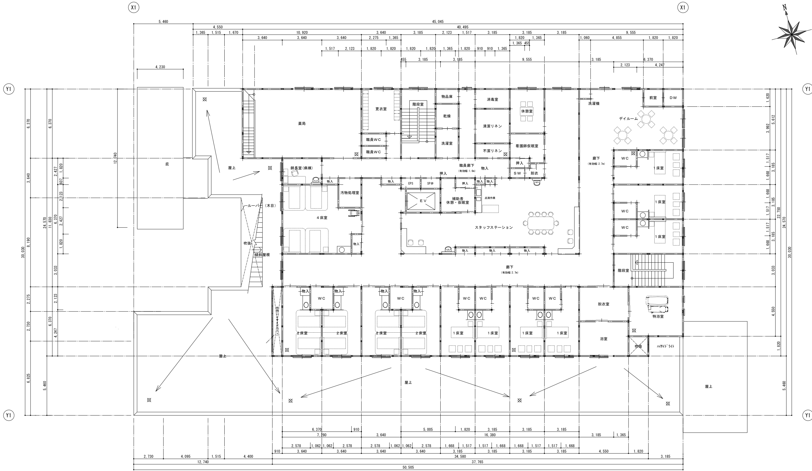
2階平面図
